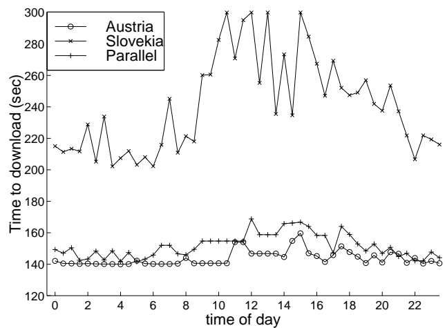
(b) S = 763 KBytes, B = 30 , M = 2 .
