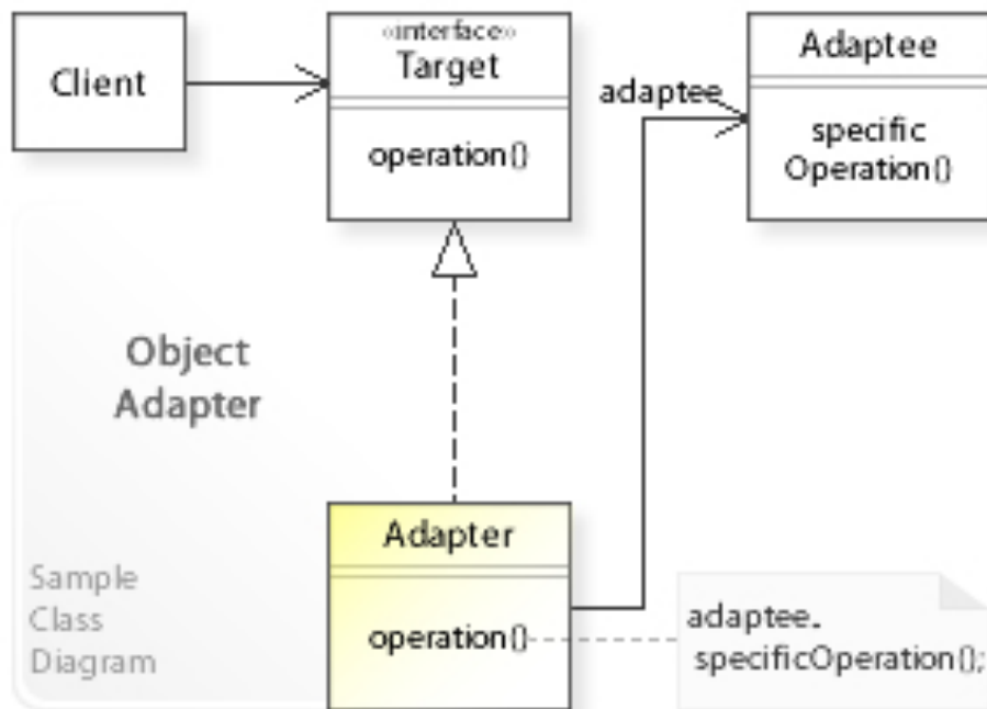
Oggetto adapter
