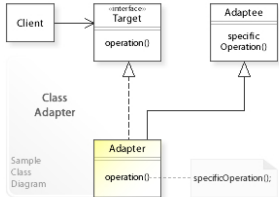
Classe adapter
