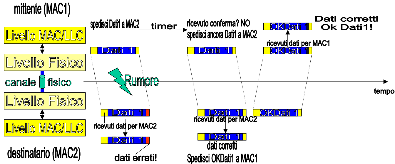
Un esempio di gestione della trasmissione a livello LLC.
